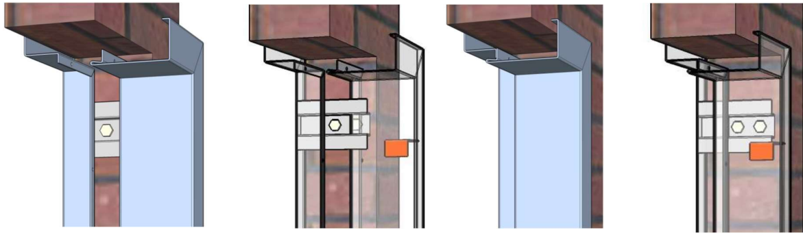
Obrázek 6. zasunutí zadního dílu zárubně do předního dílu zárubně
