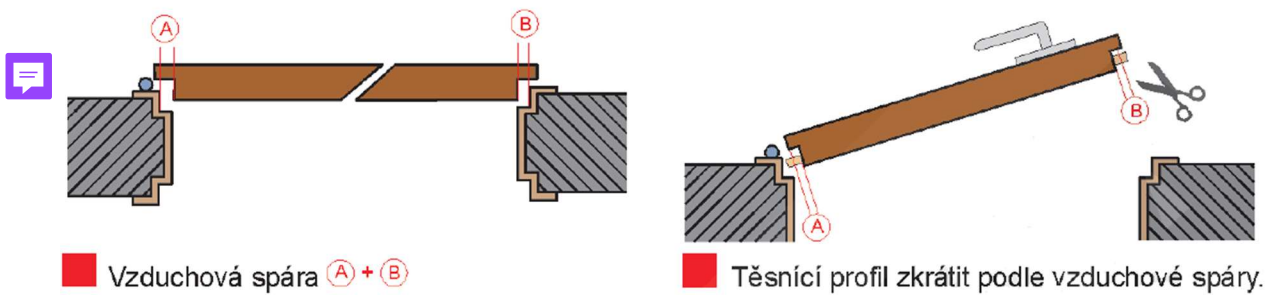
Obrázek 7. – Zkrácení těsnění padací lišty
